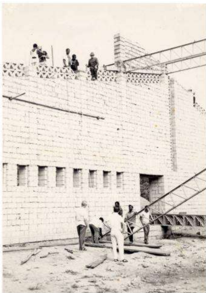
1972 Kitutu : Ferrari pose les charpentes de l'église
